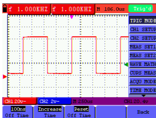
figure45:Trigger Holdoff
