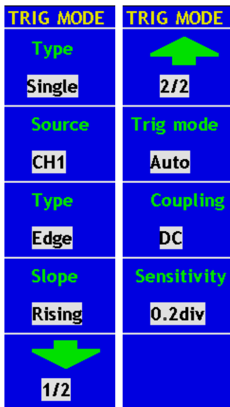
Fig. 27 Edge Trigger Menu
